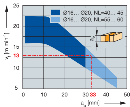
Diagramm zur Ermittlung der Vorschubgeschwindigkeit v_f in Abhängigkeit von der Nuttiefe a_p , D 16 - 20 mm
