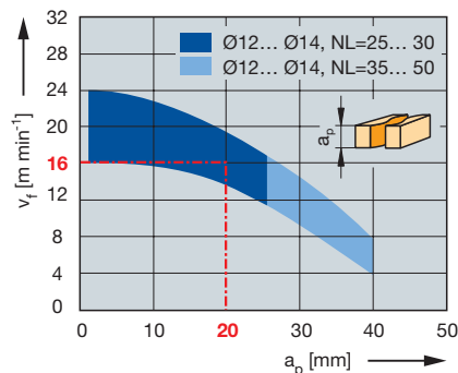
Diagramm zur Ermittlung der Vorschubgeschwindigkeit v_f in Abhängigkeit von der Nuttiefe a_p , D 12 - 14 mm
